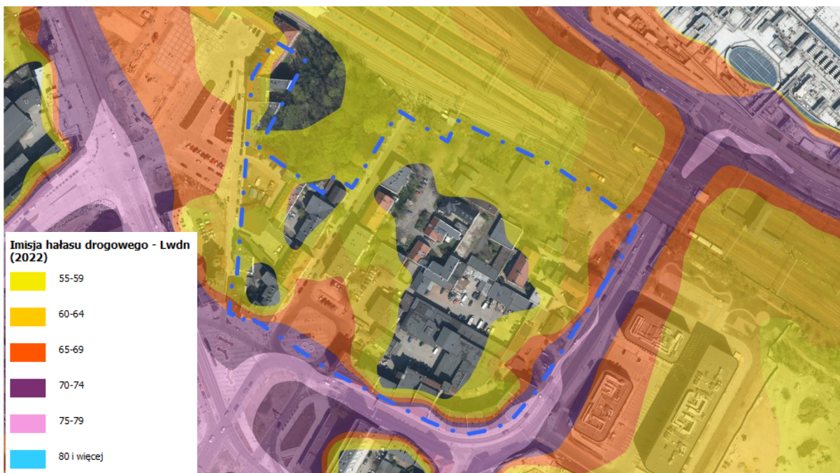
Rys. 6. Fragment strategicznej mapy hałasu dla Miasta Gliwice. Imisja hałasu drogowego L DN . Źródło: Urząd Miejski w Gliwicach, pma.gliwice.eu
