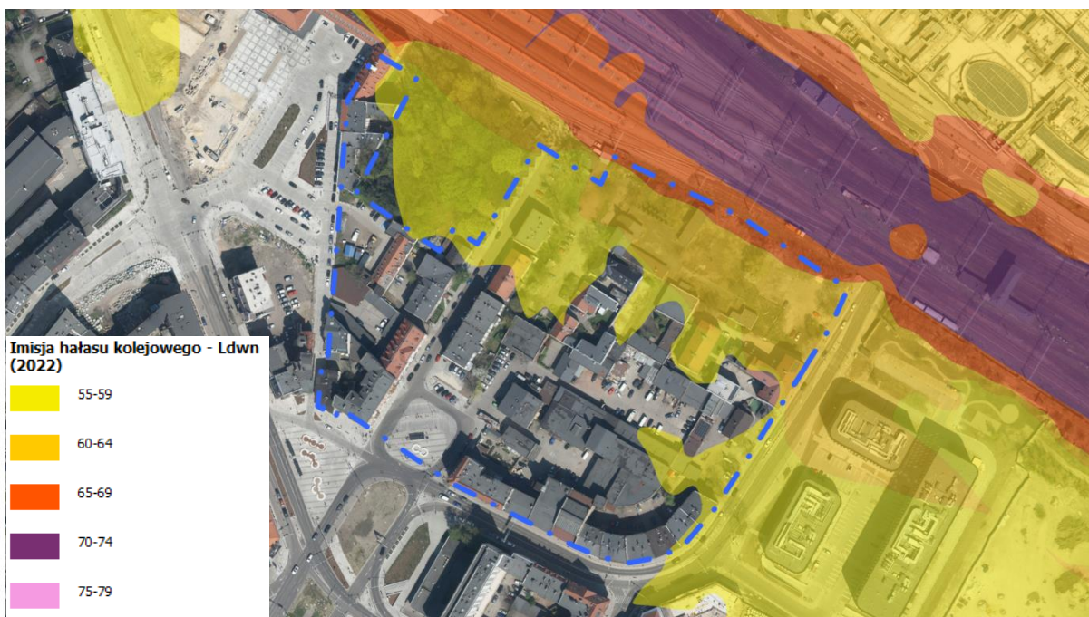
Rys. 7. Fragment strategicznej mapy hałasu dla Miasta Gliwice. Imisja hałasu kolejowego L DN . Źródło: Urząd Miejski w Gliwicach, pma.gliwice.eu
