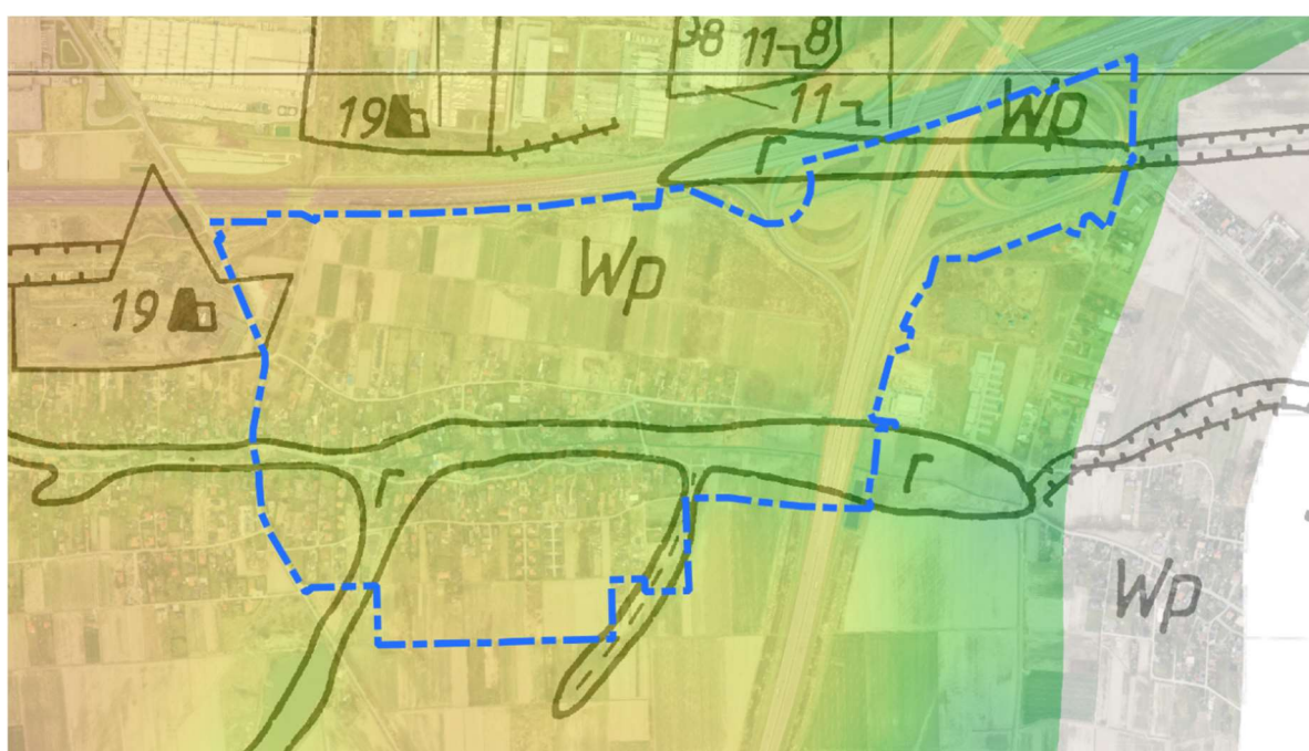
Mapa form geomorfologicznych w skali 1:25 000
