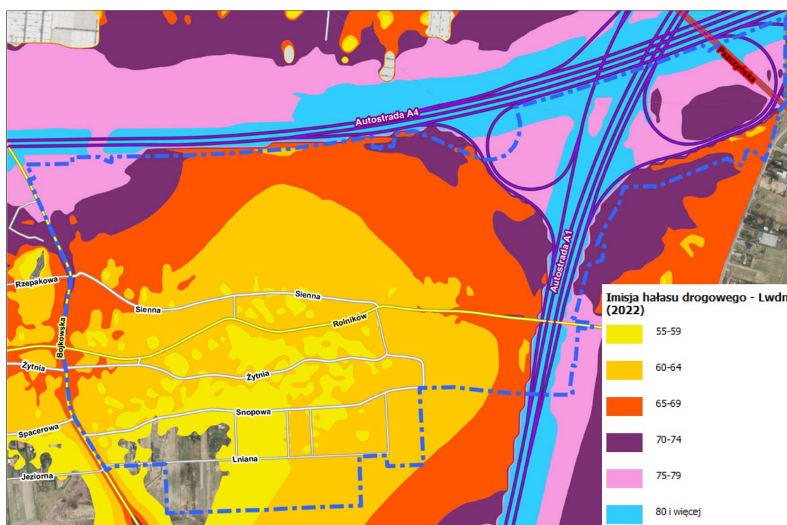
Rys. 7. Fragment strategicznej mapy hałasu dla Miasta Gliwice. Emisja hałasu drogowego L_{DWN} w dB.
