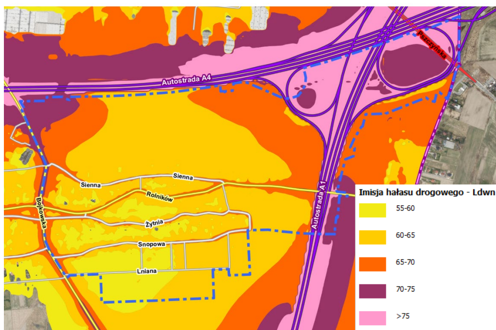
Rys. 7. Fragment mapy akustycznej dla Miasta Gliwice. Imisja hałasu drogowego L_{DWN} w dB.
